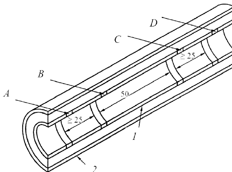
А и D - токовые электроды; В и С - потенциальные электроды; 1 - экран по жиле; 2 - экран по изоляции
