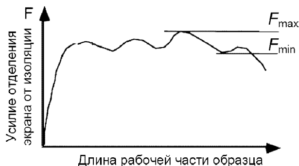
Рисунок 2. Усилие отделения электропроводящего экрана от изоляции
